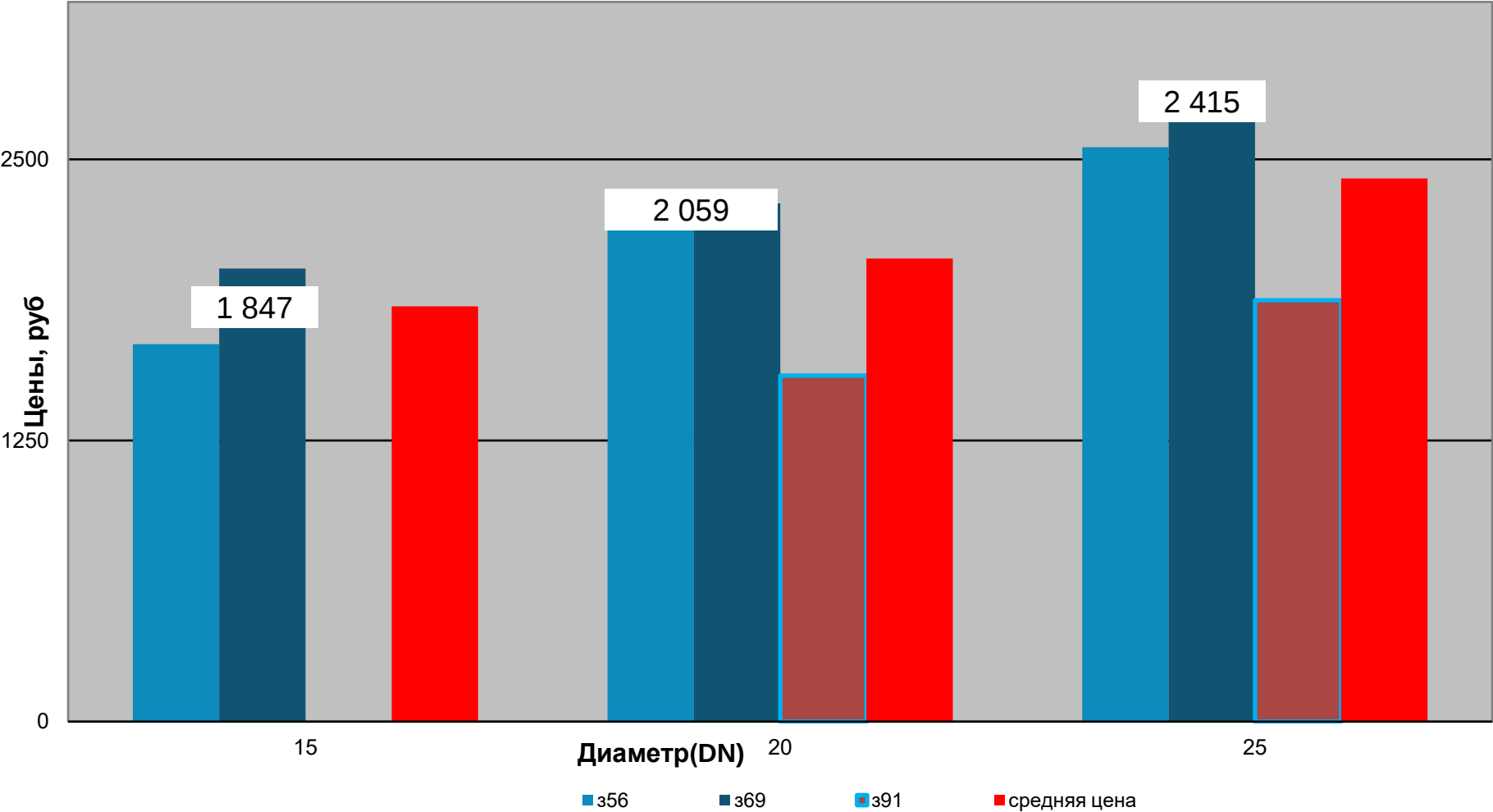
Краны шаровые, фланцевые, ст.20, PN 4,0 МПа, 1 кв. 2026 г.
