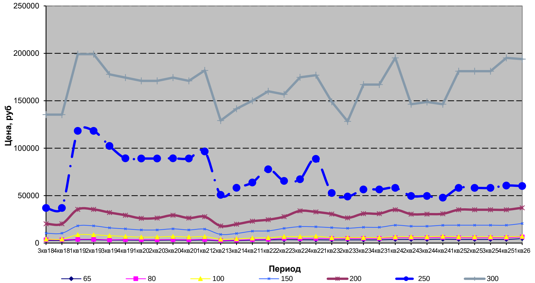
Динамика цен: краны шаровый, угл. сталь, PN 1,6 МПа
