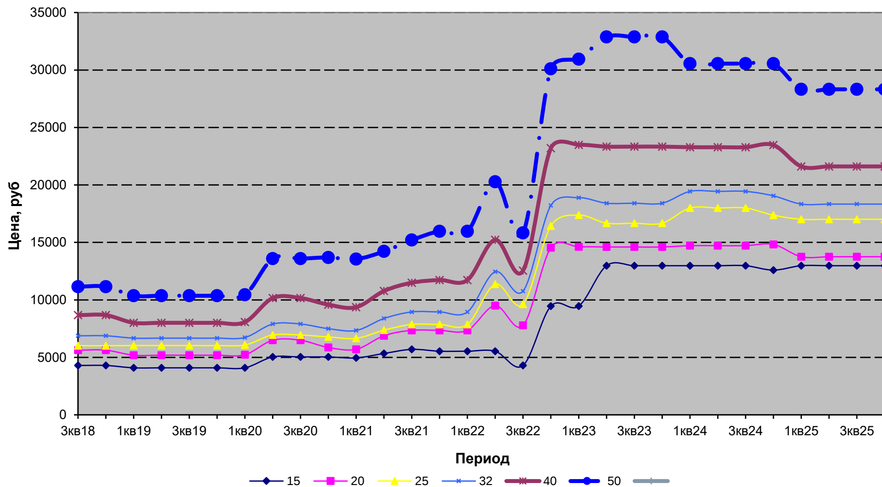
Динамика цен: краны шаровый, нерж. сталь, PN 4,0 МПа
