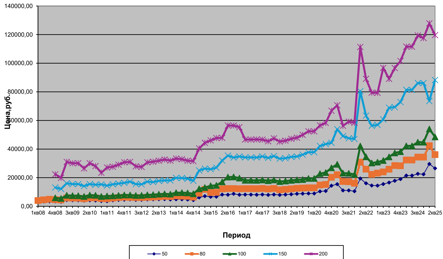
Динамика цен: задвижки стальные (30с99нж), PN 2,5 МПа
