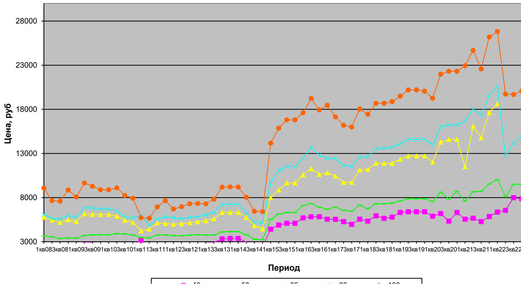
Динамика цен: Клапаны запорные из углеродистой стали (15с22нж), Pн 4,0 МПа
