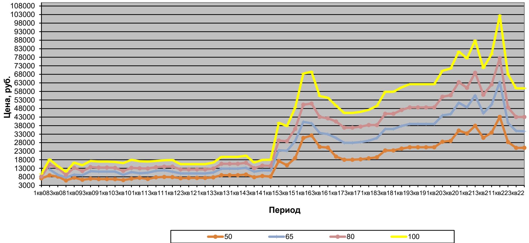
Динамика цен: Клапаны запорные из нержавеющей стали (15нж65к), Рн 1,6 МПа
